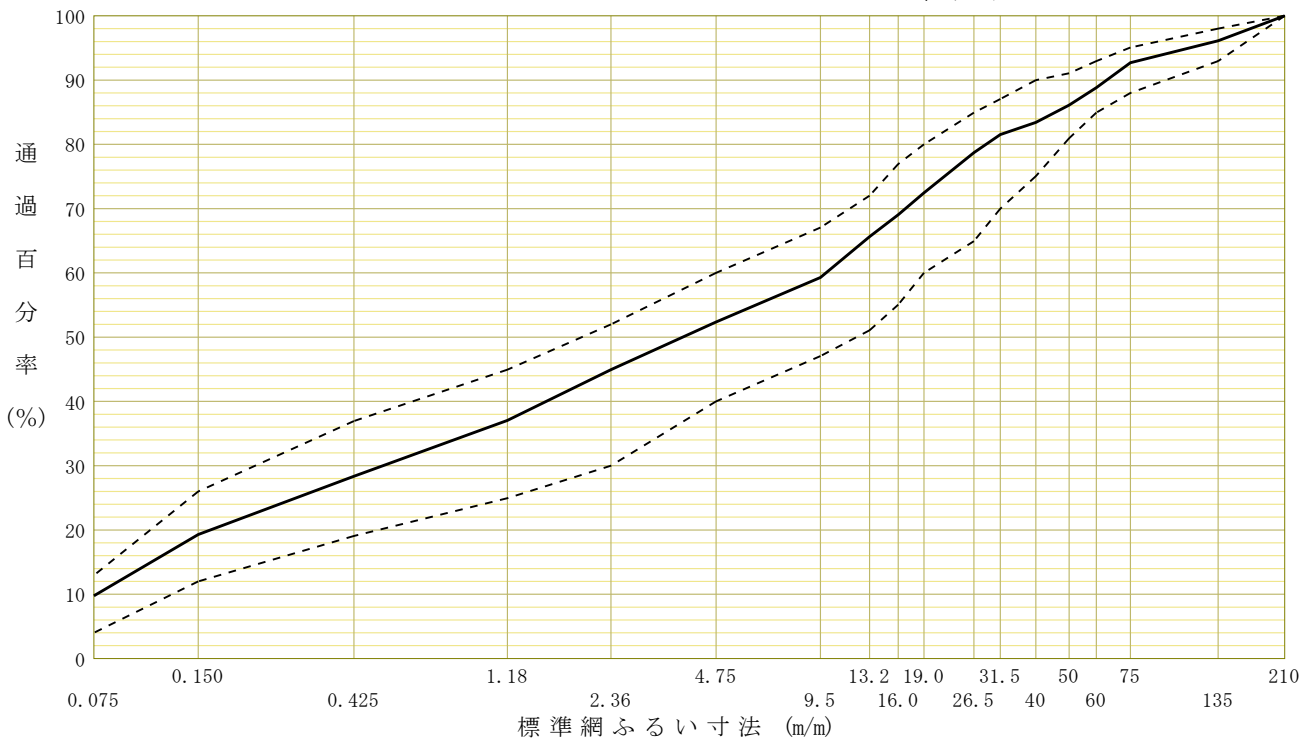
粒径加積曲線図 粗粒率 1.61
